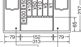
紙幣収納枚数 320枚 320枚 (目安) 【合計640枚】 ※1000円札/2000円札/5000円札/10000円札いずれも
