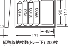
紙幣収納枚数(トレー下) 200枚 (目安) ※1000円札/2000円札/5000円札/10000円札いずれも
