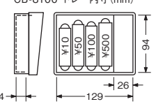
紙幣収納枚数(トレー下) 200枚 (目安) ※1000円札/2000円札/5000円札/10000円札いずれも
