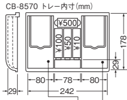
トレー外寸(コインカバー部含まず) W253×L184×H43mm (※別売なし)
