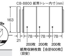
トレー外寸 W246×L120×H25mm (※別売なし) CB-8800 コイントレー内寸(mm)
