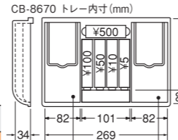
トレー外寸(コインカバー部含まず) W280×L205×H48mm (※別売なし)
