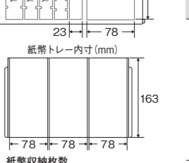
トレー外寸 W246×L120×H25mm (※別売なし) フリースペース内寸(mm)
