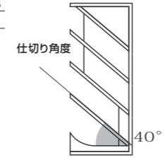
仕切り角度 40° 仕切り板に40度の傾斜がついておりペンが取り出し易い設計。
