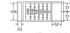
トレー外寸 W246×L120×H25mm (※別売なし)
